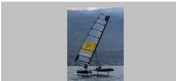
Catamaran à foils à a gréement basculant
