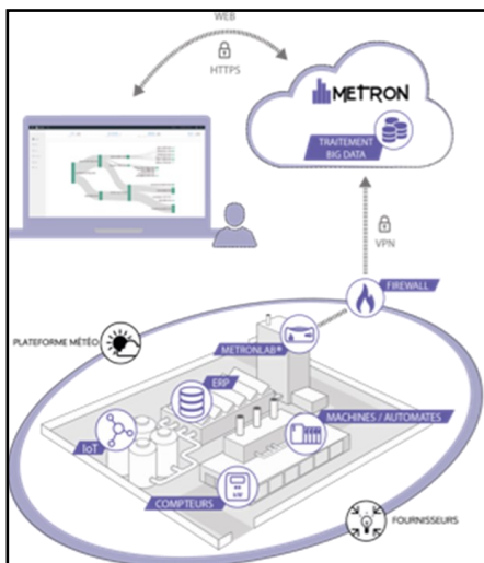
Représentation schématique du système VAF-IA
